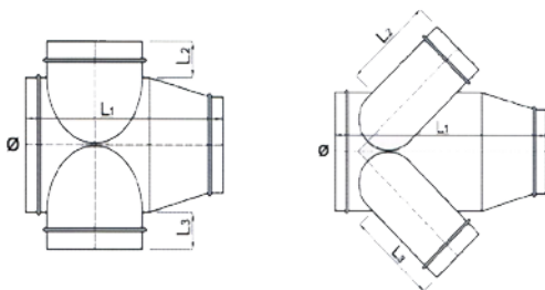
CRUZ CÓNICA
