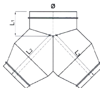
DERIVACIÓN CÓNICA
