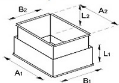
Cuello telescópico
