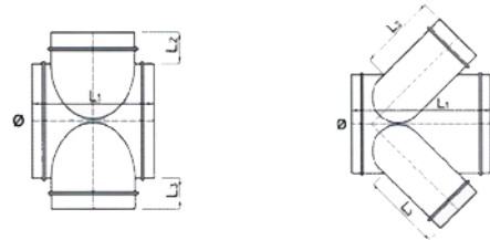
CRUZ SIMPLE
