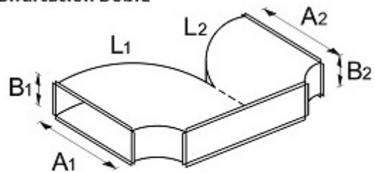
Bifurcación Doble
