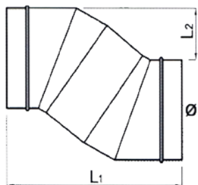
DESVÍO CIRCULAR
