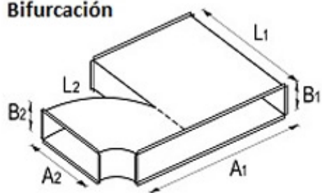
Bifurcación
